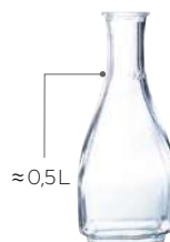
≈0,5L 0,5 L Ø M = 95 mm H = 200 mm W = 350 g 53673 A12=12
